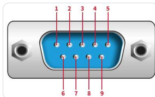
Abbildung 1 · Steckerbelegung
