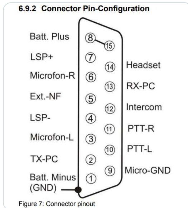
Figuur 1 · KRT2 connector pinout
