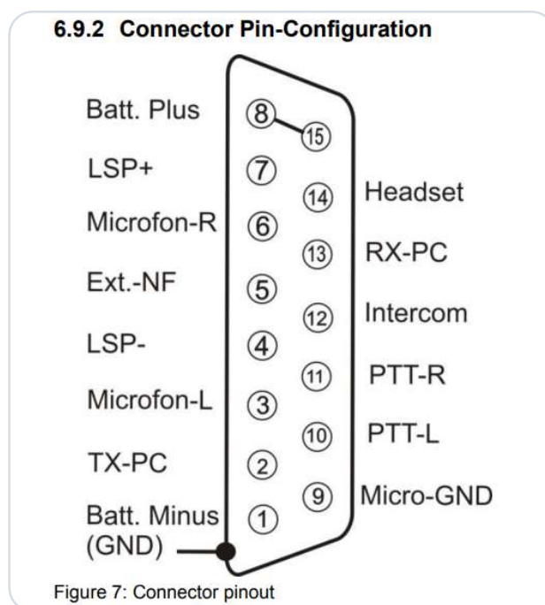
Figure 1 · Affectation des broches du connecteur KRT2
