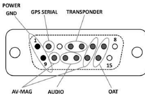
Figura 5 · Assegnazione pin del connettore AV-30
