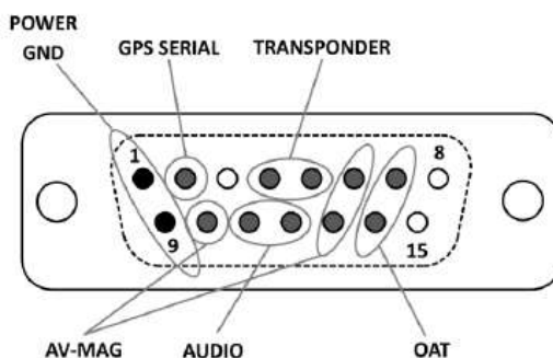
Figure 5 · Affectation des broches du connecteur AV-30
